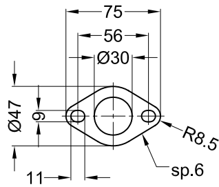
Vista "B" Flangia "45D"
